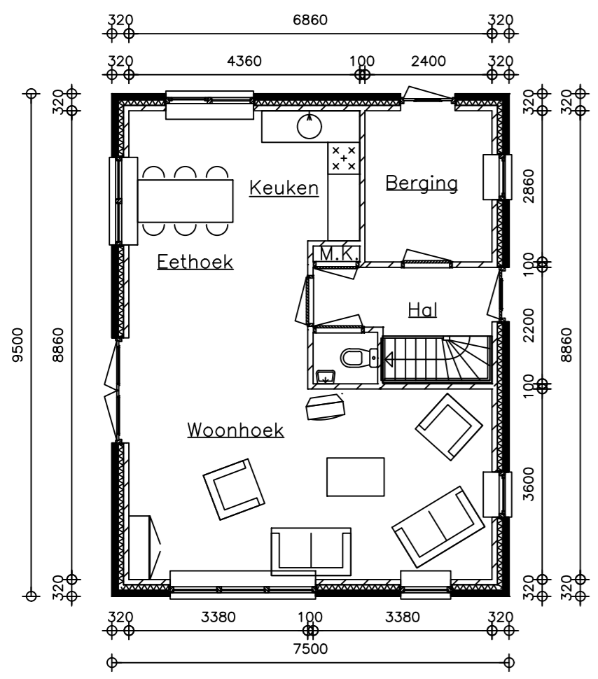
Begane grond
