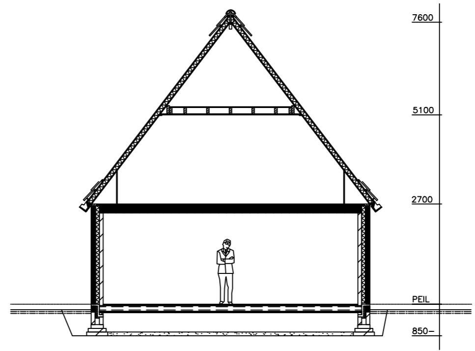
Doorsnede
