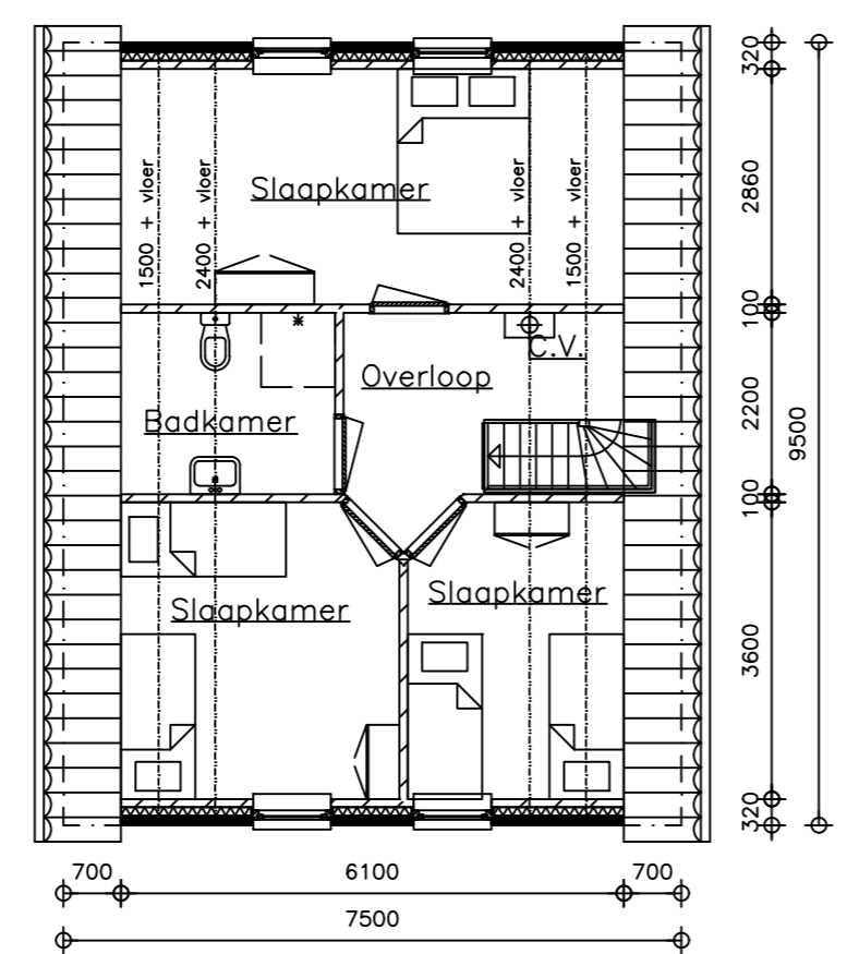
Verdieping
