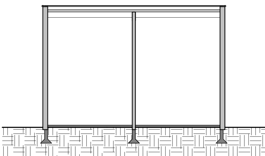
Doorsnede A
